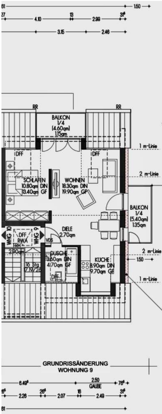
Grundriss DG
